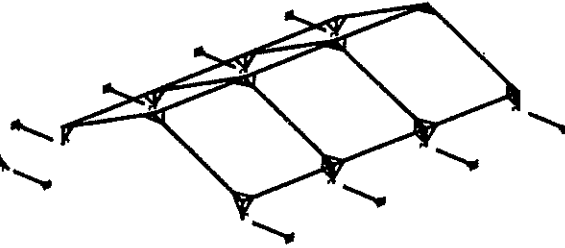
② - Assembler le toit
