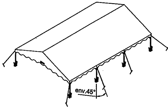
⑥ - Ancrages des pieds et haubannages
